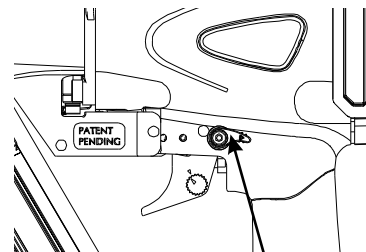
Bouton antidéclenchement (B)
