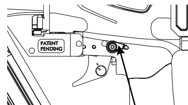
Botón de bloqueo de activación de disparos (B)
